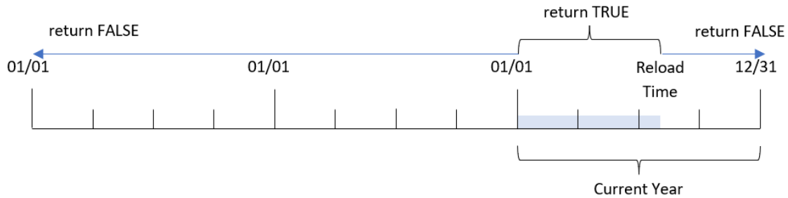
yeartodate() 函數的範例圖表
