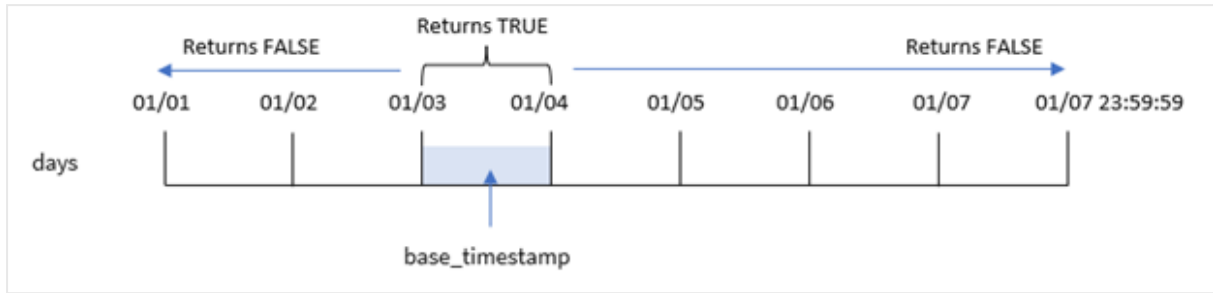
inday 函數的圖表
