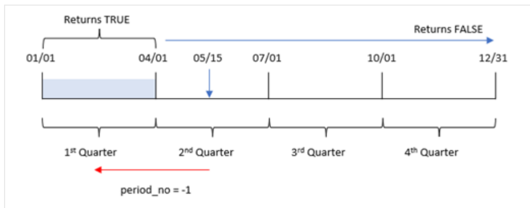
Диаграмма функции inquarter() с базовой датой 15 мая
