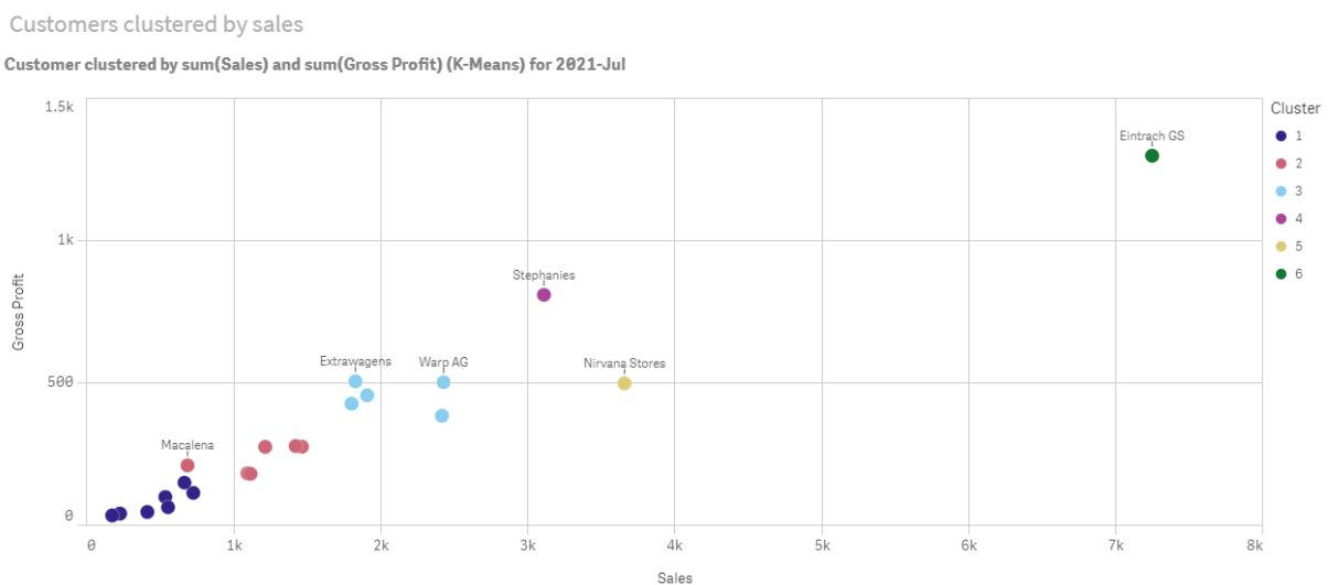
Gráfico de dispersión de k-means tras las modificaciones
